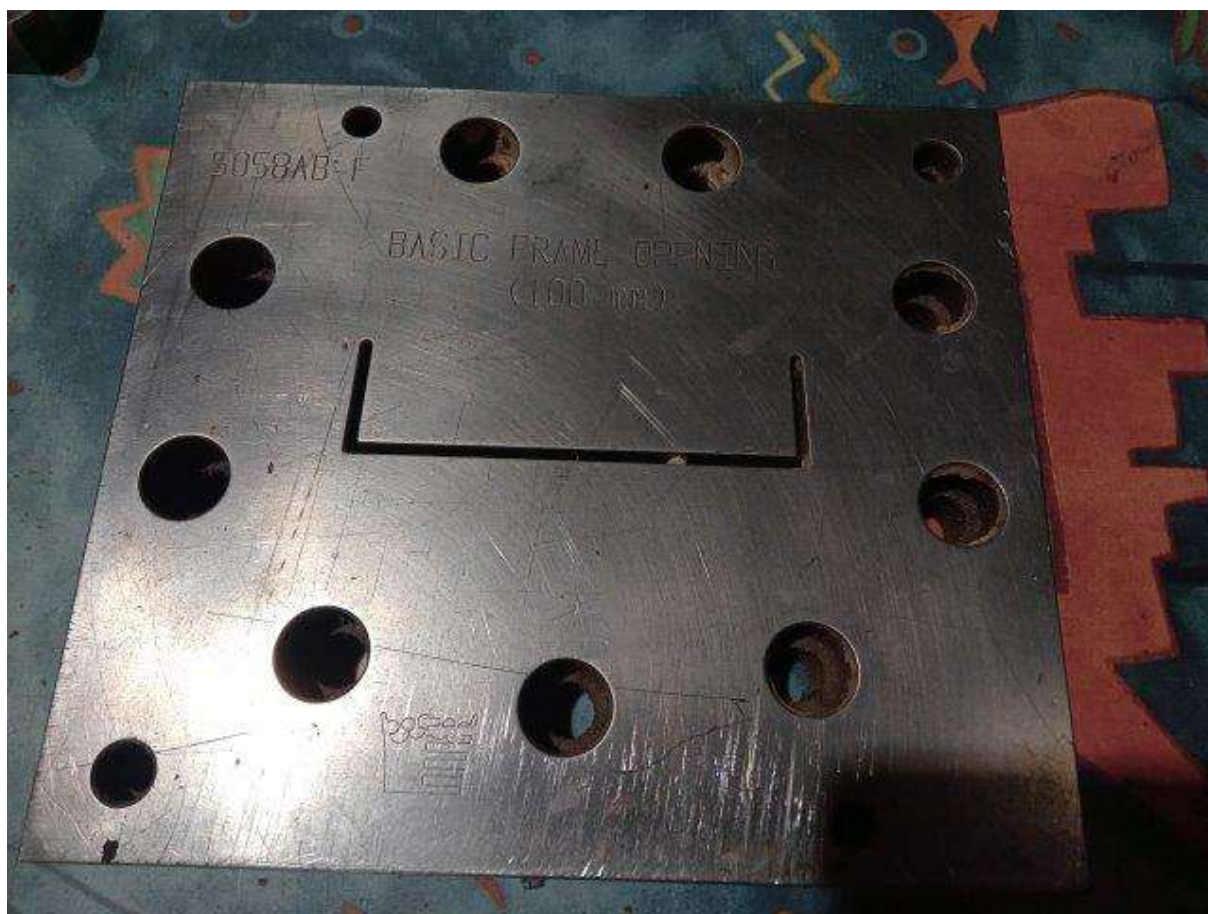
wanna chłodząco-kalibrująca
