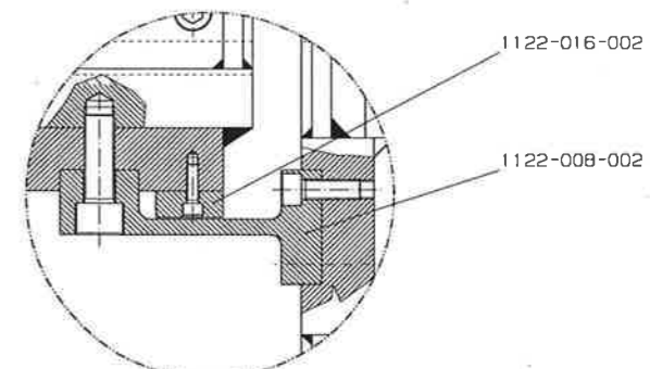
DETTAGLIO -A- SCALA 1:2
