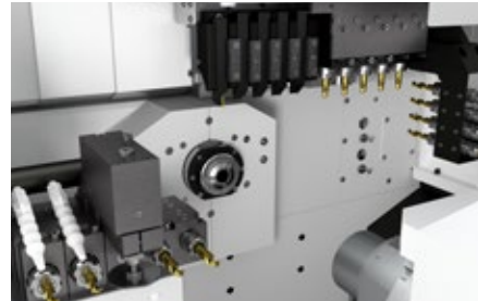
5 linear axis
