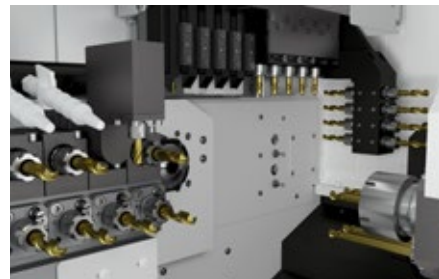
6 linear axis**
