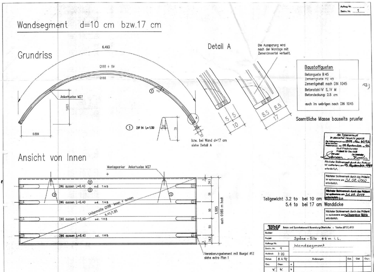
Abb. A.4 Wandsegment der im Jahre 2005 gültigen Typenstatik
