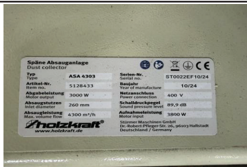
Ansicht Typschild Absauganlage
