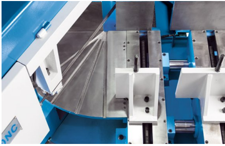
Schnittwinkelverstellung 0° - 45°
