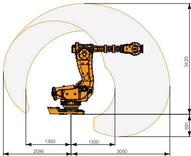
IRB 7600-340/2.8
