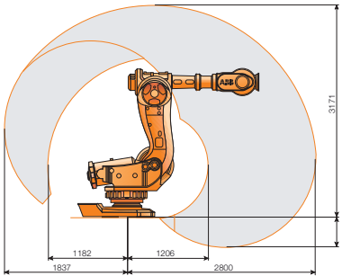
IRB 7600-340/2.8
