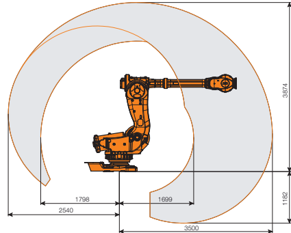
IRB 7600-150/3.5
