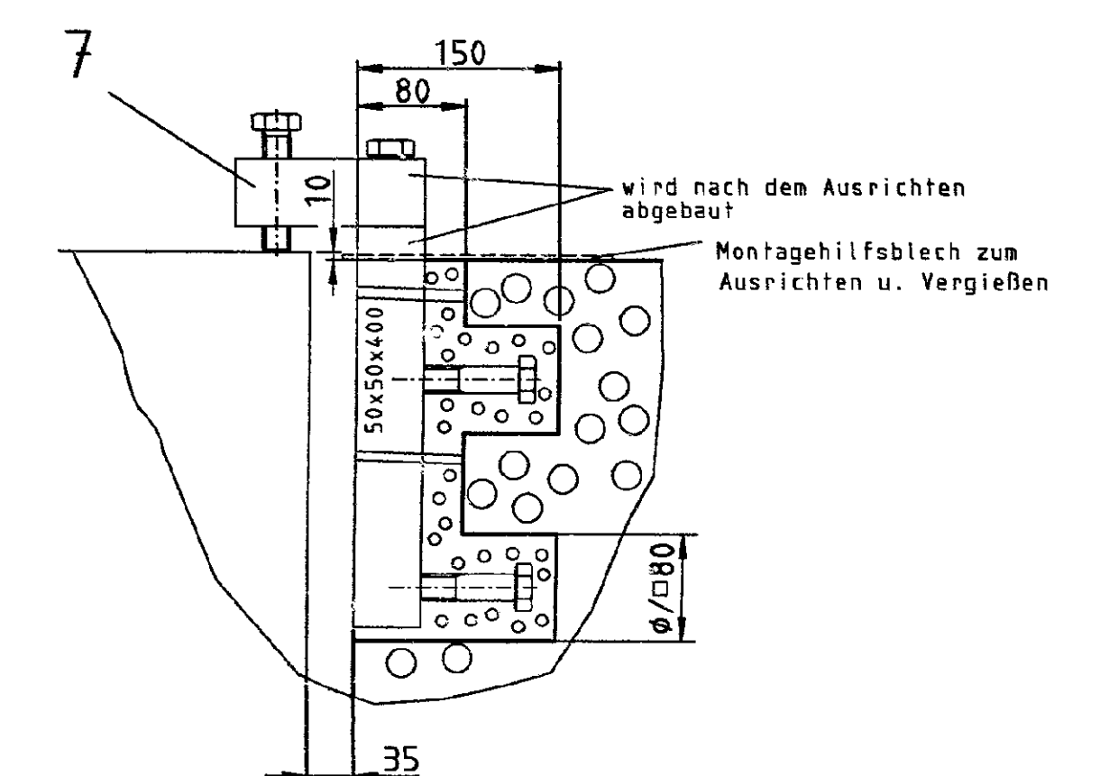
Schnitt E - E M 1:5
