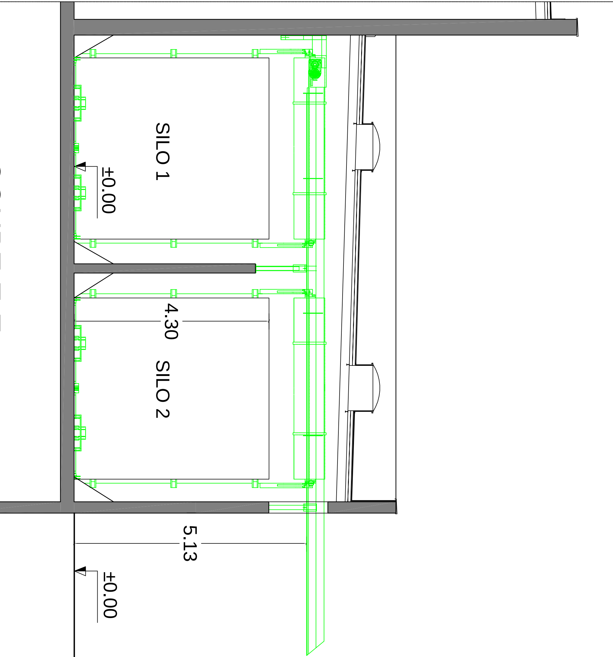
COUPE E-E
