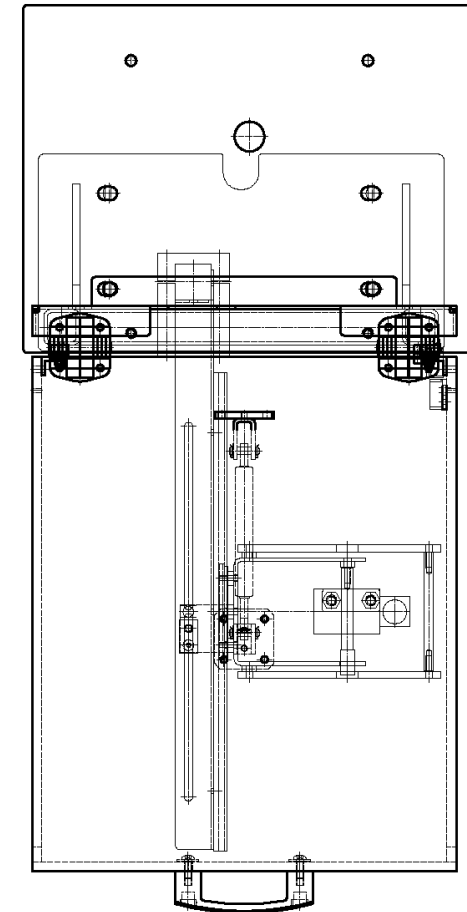
Draufsicht Acrylschutzhaube
