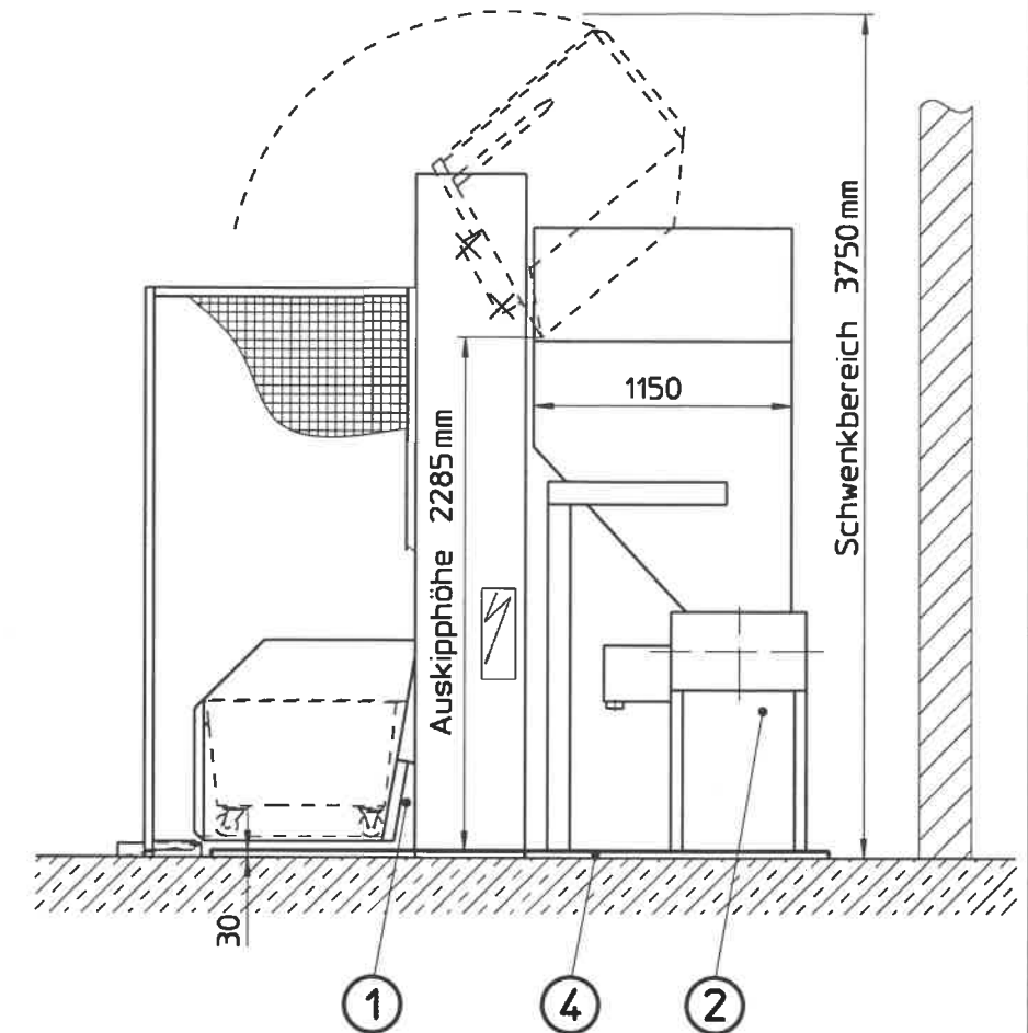
Schnitt A-A
