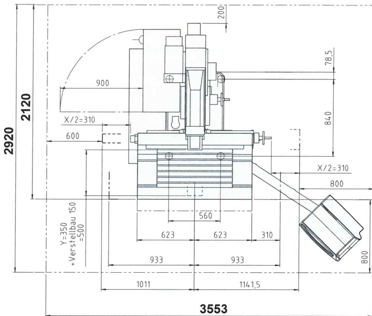
Abbildung 3: Aufstellplan FPS620M-NC
