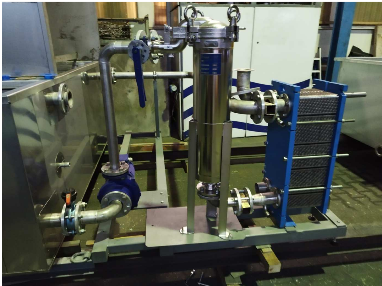
Umwälzpumpe mit Beutelfilter und Plattenwärmetauscher mit neuen Dichtungen
