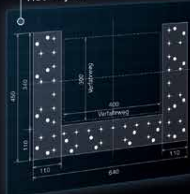
Tischlayout
