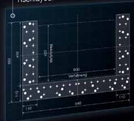
Tischlayout
