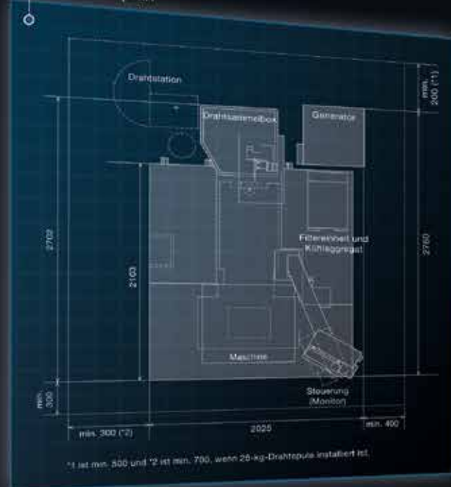
Maschinenplan
