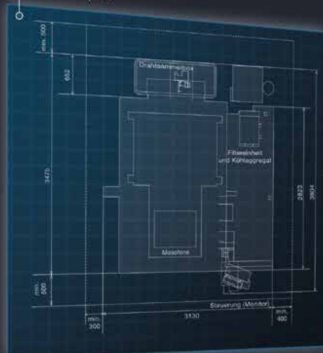
Maschinenplan
