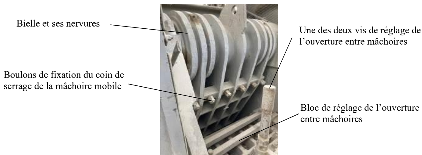
Fig. XI Vue paroi latérale de la carcasse, la bielle, le bloc arrière de réglage de l'ouverture entre mâchoires, une des deux vis de réglage au pas trapézoïdal et sa protection
