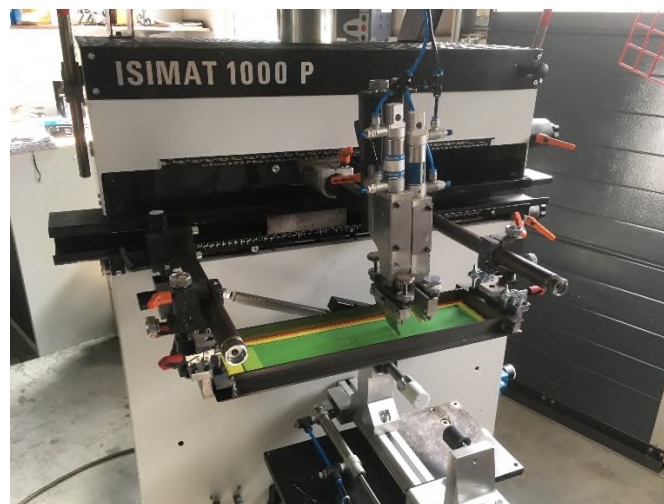
Halbautomatische Siebdruckmaschine für Flach / Runddruck
