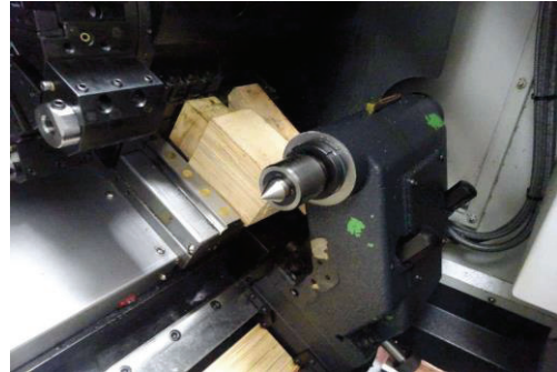
Ansicht Reitstock
