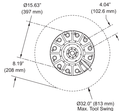
VDI Turret
