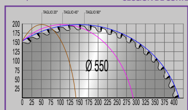
TRGSI Ø 550 SECCIÓN DE CORTE
