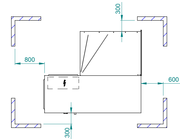
SPAZI DI INSTALLAZIONE / CLEARANCES
