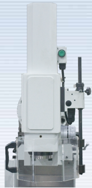
Spindelstock mit hydraulischer Werkzeugklemmung
