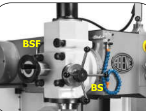
SPINDELKOPFTYPEN BS: Bohrspindel, Pinole mit 75 mm Hub, Bedienung über Handhebel BSF: Handrad für Feinvorschub 3mm / Umdrehungen Option: digitale Winkeldarstellung
