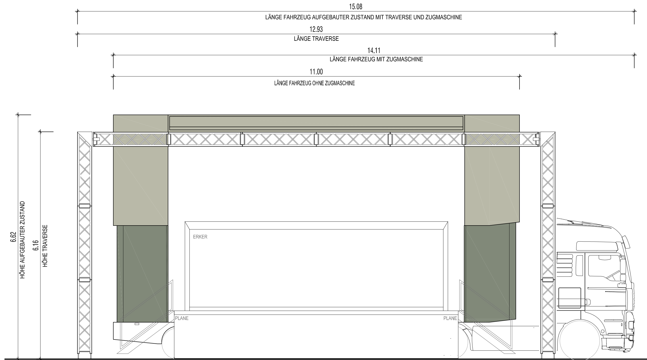
ANSICHT 1 -AUFGEBAUT-
