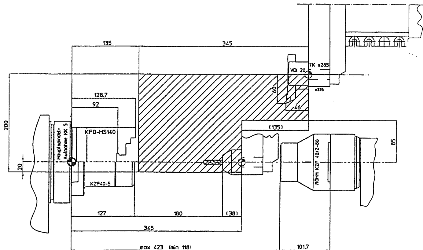
Bild2- 3:Arbeitsraumplan
