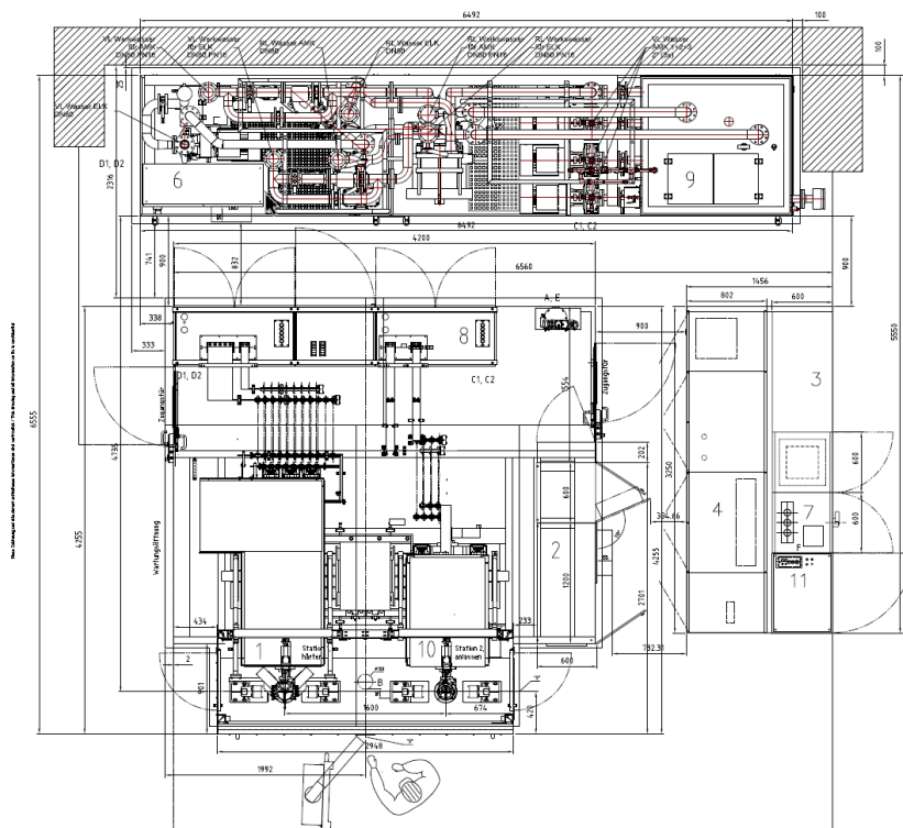
Aufstellfläche ( floor space)
