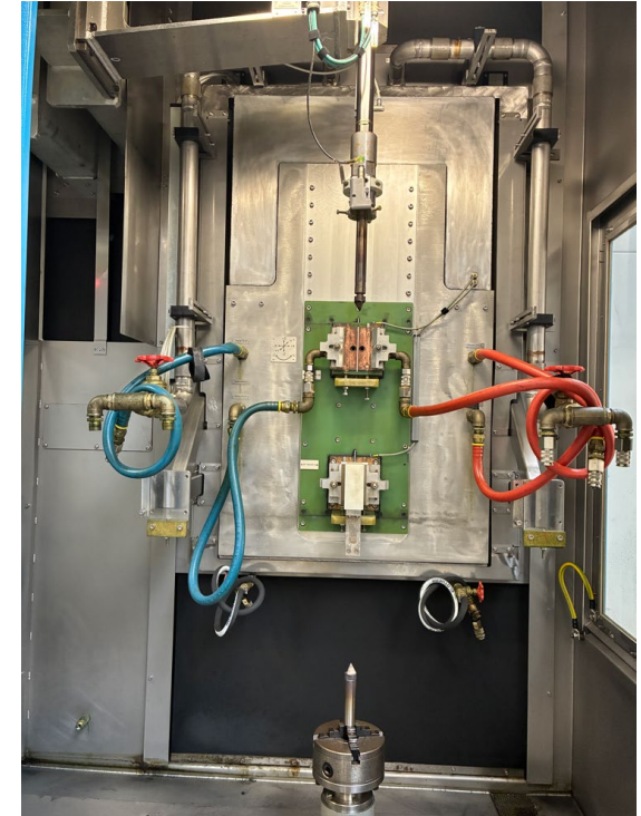
Maschine-Arbeitsraum ( workspace of machine )
