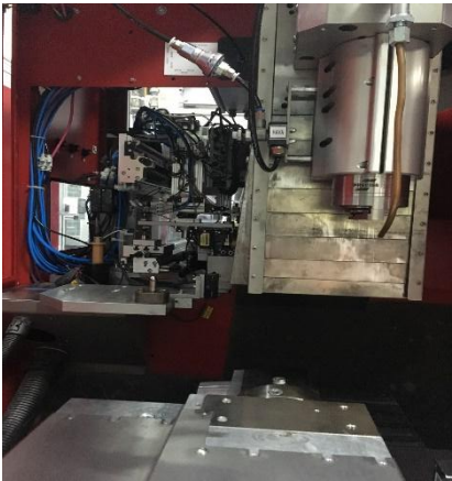
Arbeitsraum (workspace of machine)
