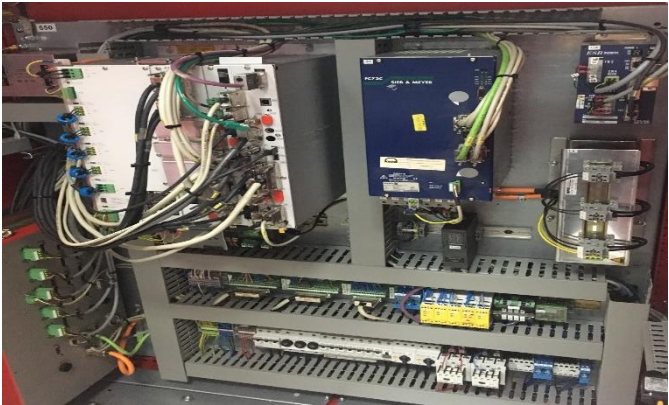
Steuerung (control unit)
