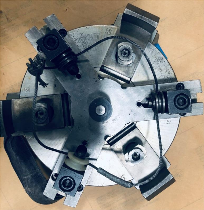
Kraftspanfutter KFD-HSmB 250/3
