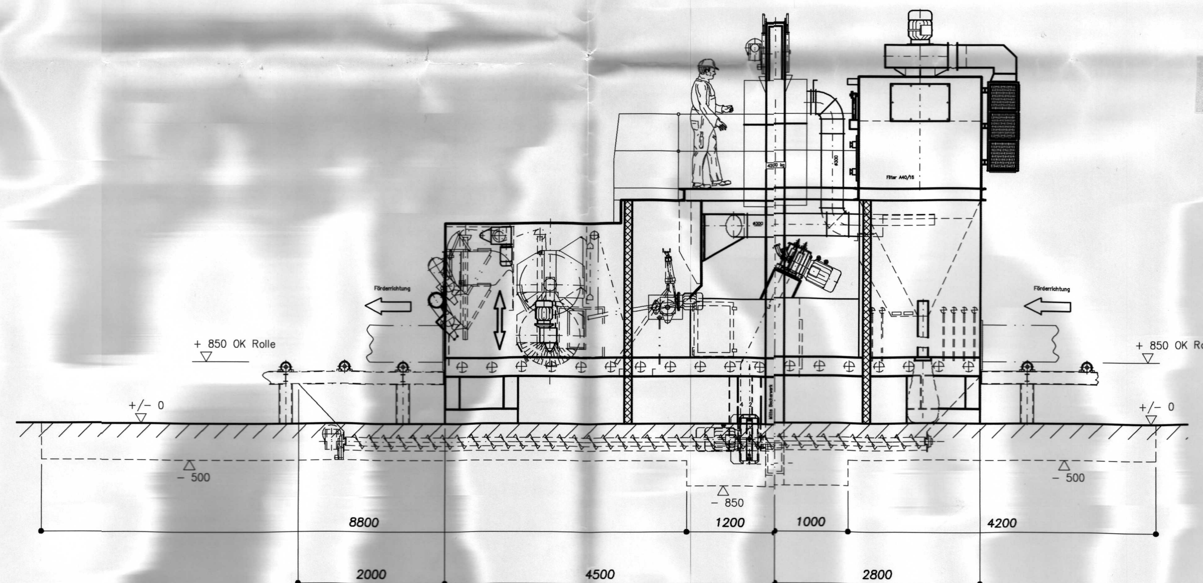
Schnitt B-B M.: 1:50
