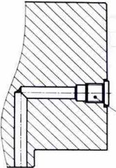
Teilschnitt im Zylinderdeckel
