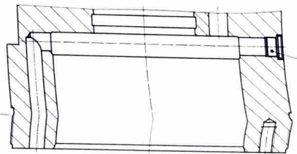
Teilschnitt im Zylinderrohr
