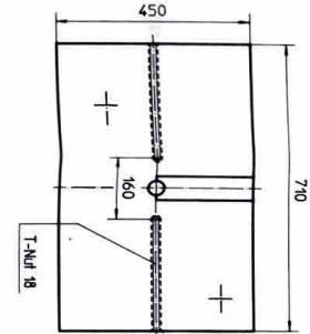
Pressenstößel M 110 710
