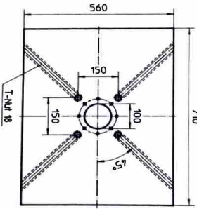
Pressentisch M 110 710
