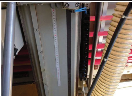
Ansicht Vertikalführung
