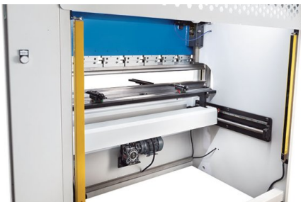
Die Rückseite ist durch Lichtvorhänge geschützt
