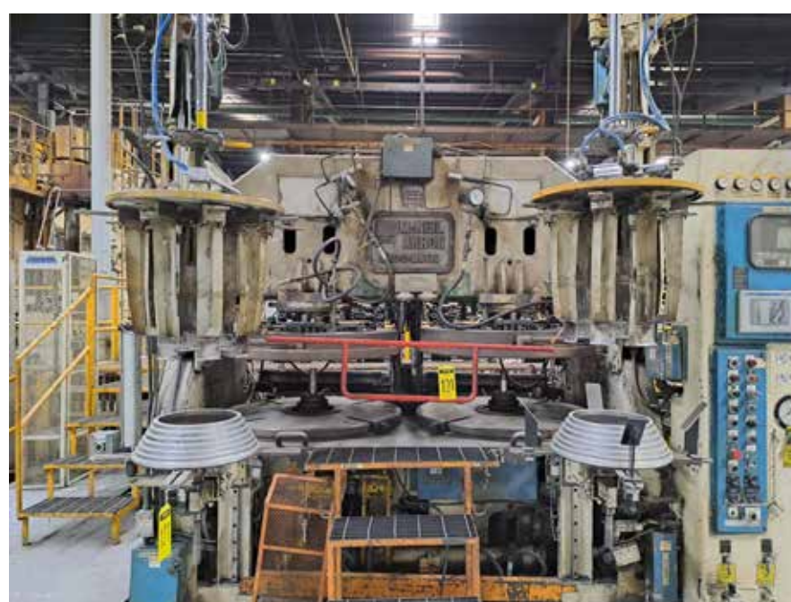
Lote 121: Prensa de Vulcanización a vapor Marca MC NEIL AKRON, Modelo 300-4215PM-16, Serie BP708555277, con presión máx de 300,000 lbs, Fuerza de Cierre Mecánico: 300 Toneladas, Tamaño Nominal de Platos: 42"
