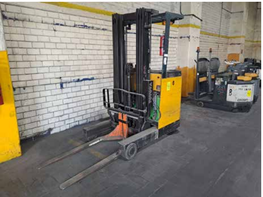
Lote 44: Montacargas Eléctrico Tipo Hombre Parado Marca Toyota, Modelo 7FBR15, Año 2006 , Altura Máx 5 Mts , Capacidad 1,400 Kg, Voltaje 48 V.
