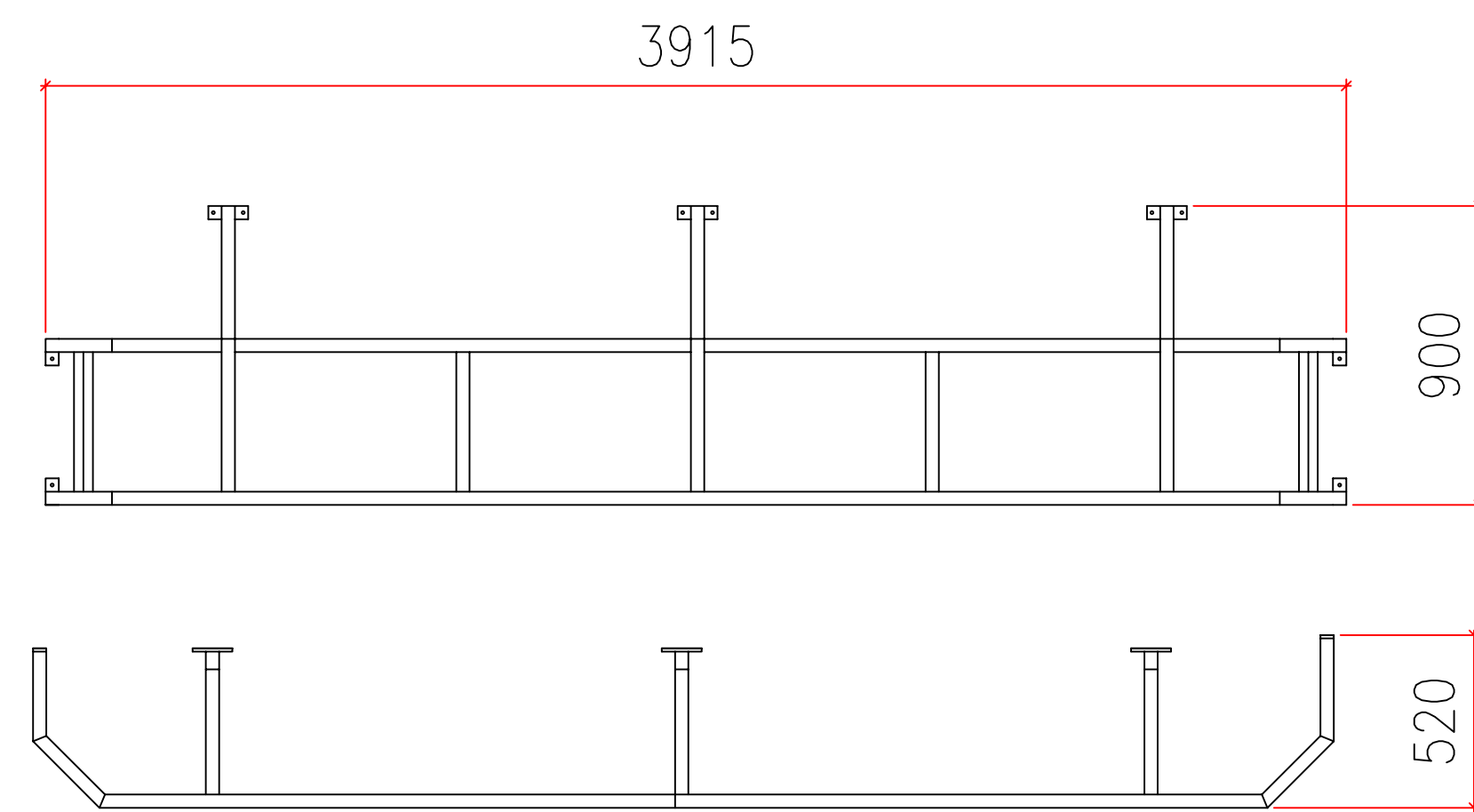
PROTEZIONI LATO DESTRO PROTECTIONS RIGHT SIDE KG. 40
