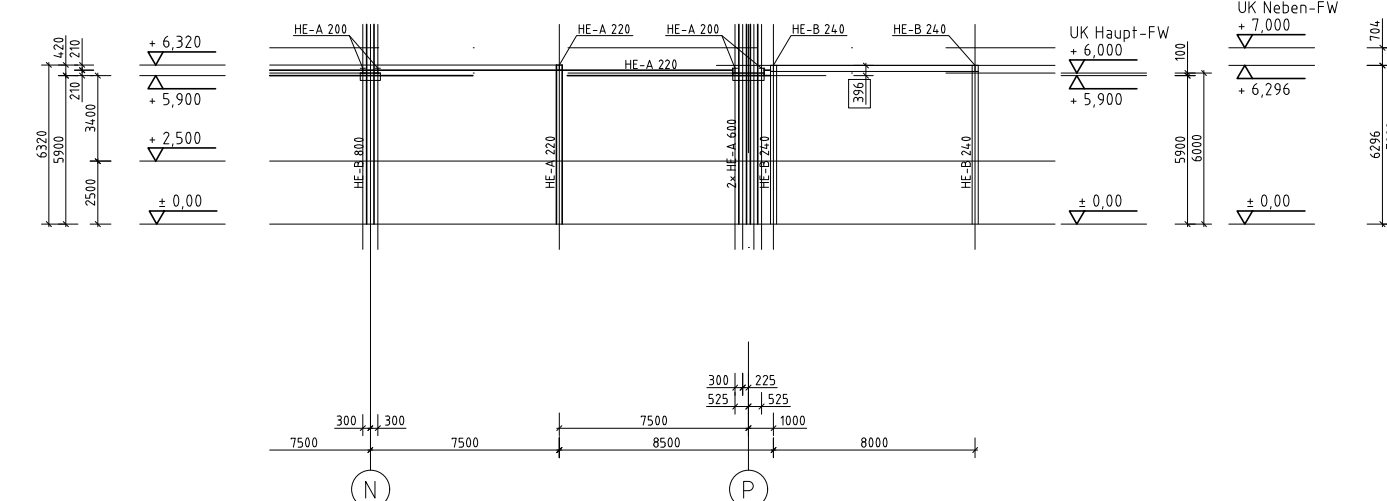
Regel - Längsschnitt - Übergabe Achse 6
