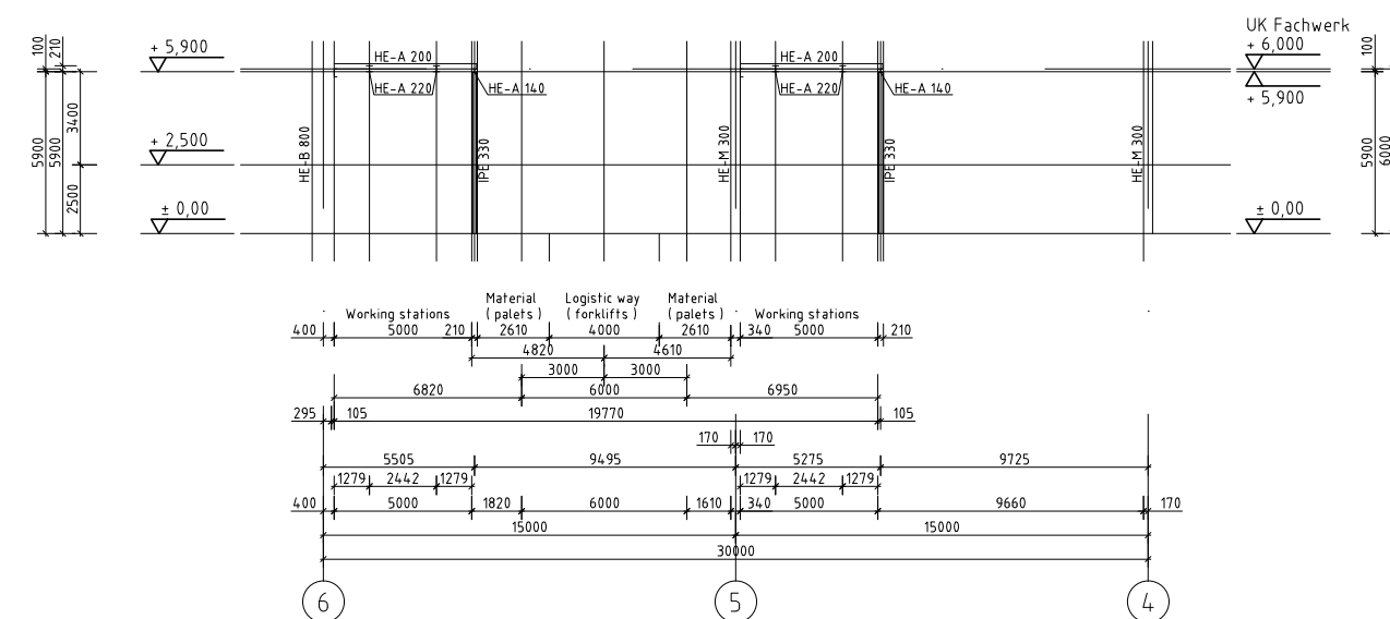
Regelschnitt mit Bestandsstützen
