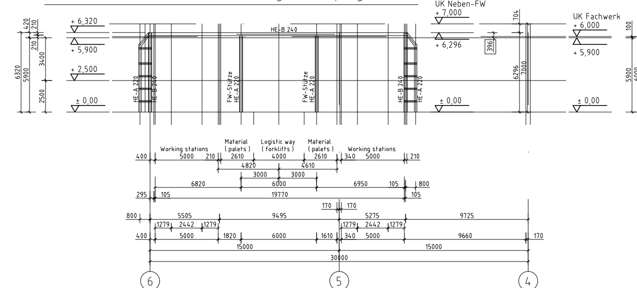
Ansicht von Reihe P in Richtung N im Spiegelbild
