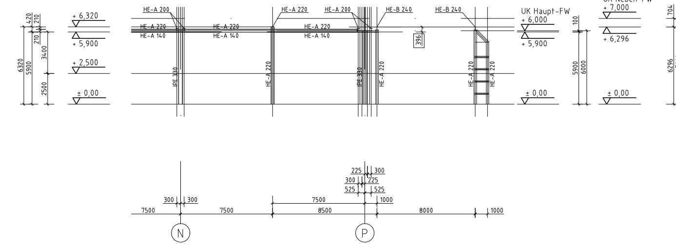
Regel - Längsschnitt - Übergabe
