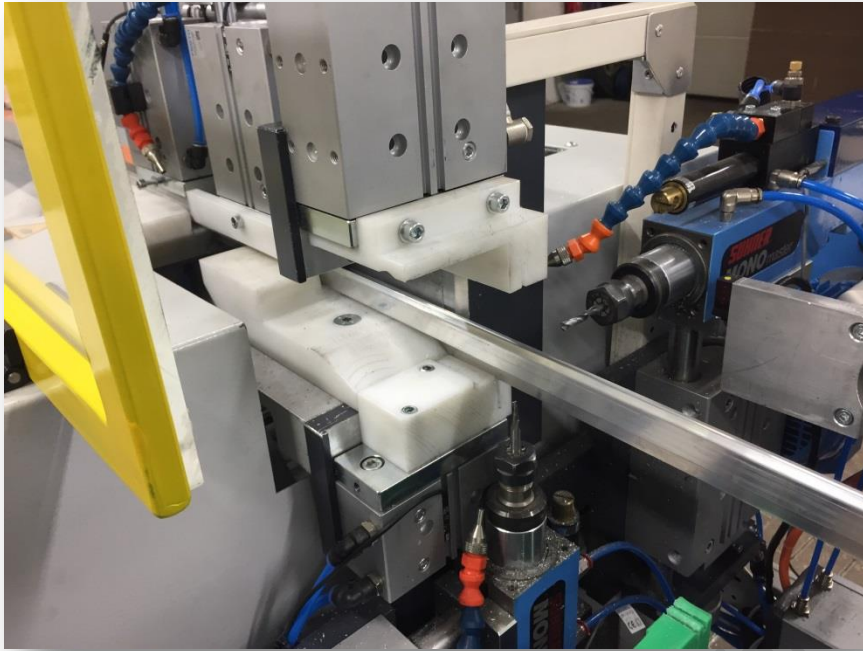
Horizontale und vertikale Bohr-/Fräseinheiten incl. Profilspannbacken
