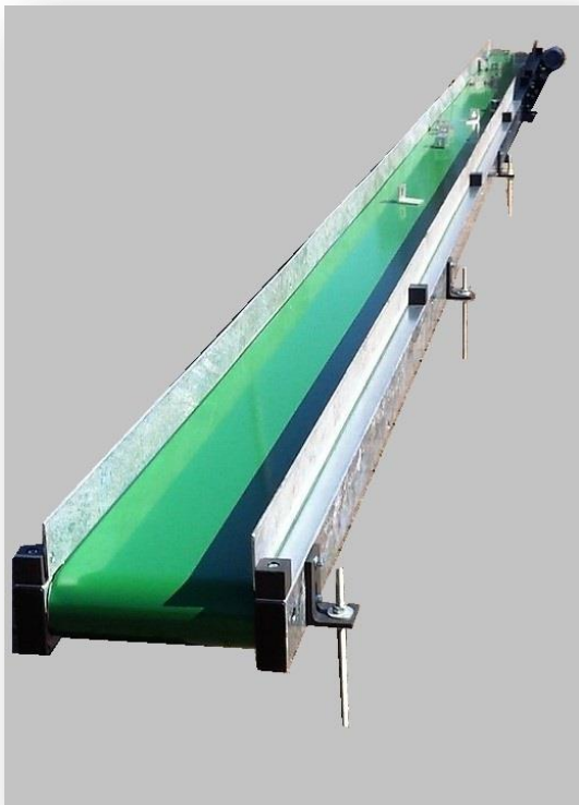
Späne-Transportband (Länge bis 7 Meter)
