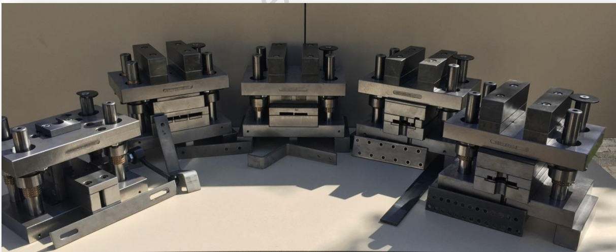
Werkzeuge für den Solaranlagenbau (Biegen/Lochen/Langlöcher/Räumen/etc.)
