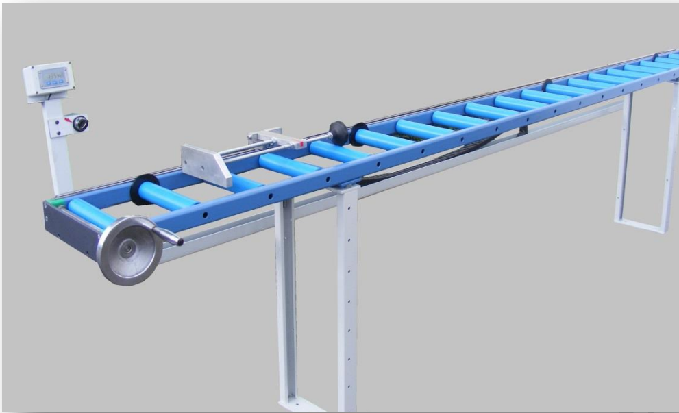
Rollenbahn-Längenanschlag mit Handkurbel und Digitalanzeige
