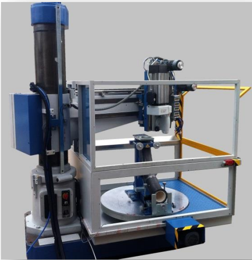
Schleifmaschine zur Bearbeitung von Keramikrohren
