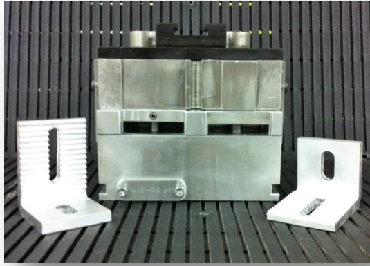
Langlochwerkzeug für Halter Solarpaneele
