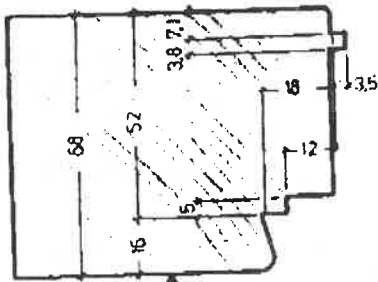
FK - Flügel Kontor - Null-Ø 314 mm Bestell-Nr. SH 95 TM 14 01
