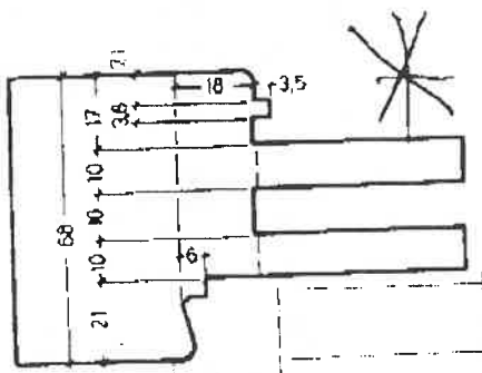
FZZ - Flügel Zapfen Zusatzfräser für 2fach Zapfen solo auf Büchse Bestell-Nr. SH 95 TM 13 01
