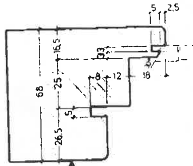
FÜD - Flügel Überschlagsrichtung auf Büchse Bestell-Nr. SH 95 TM 17 02
