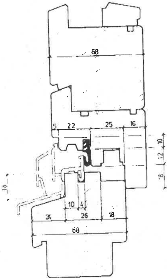
FAso - Flügel Außen seitlich und oben mit Getrieberut Bestell-Nr. SH 95 TM 02 02
