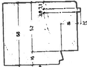
FIG - Flügel Innen Gegenprofil - Null-Ø 125 mm Bestell-Nr. SH 95 TM 15 01
