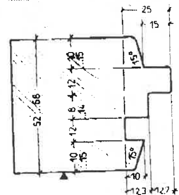
RAU - Rahmen Außen unten ohne Fügebearbeitung Bestell-Nr. SH 95 TM 26 03
