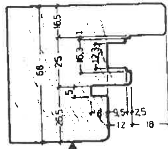
FAso - Flügel Außen seitlich und oben mit Getrieberut Bestell-Nr. SH 95 TM 02 02
