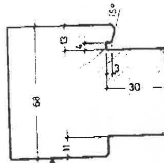
RAU - Rahmen Außen unten ohne Fügebearbeitung Bestell-Nr. SH 95 TM 18 01
