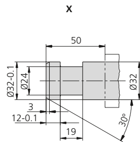
Auswerferbolzen
