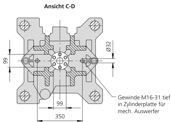
Ausdrehung im Werkzeug nur, wenn kurzer Anguss gewünscht wird
