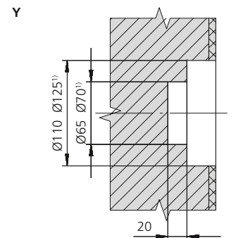
Maße für Duroplastwerkzeuge
