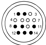
AMP-Steckdose
