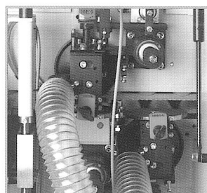
Radienziehklinge
