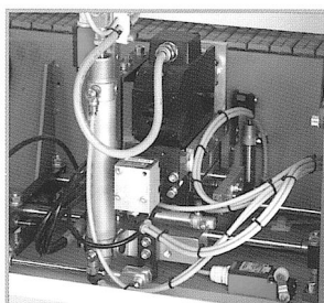
Eckenfräse
