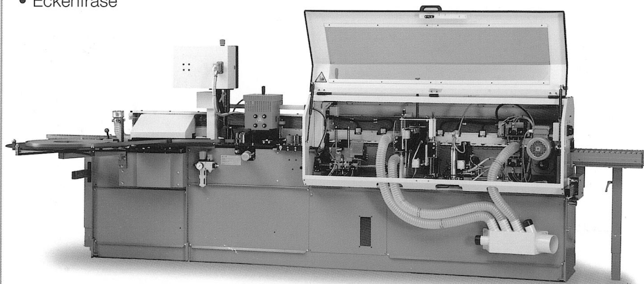
AKV 3003 DK-F
