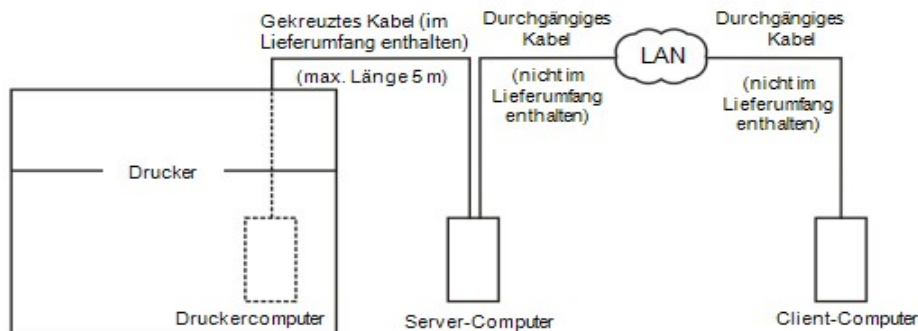
Abbildung 5 Netzwerkinstallation
