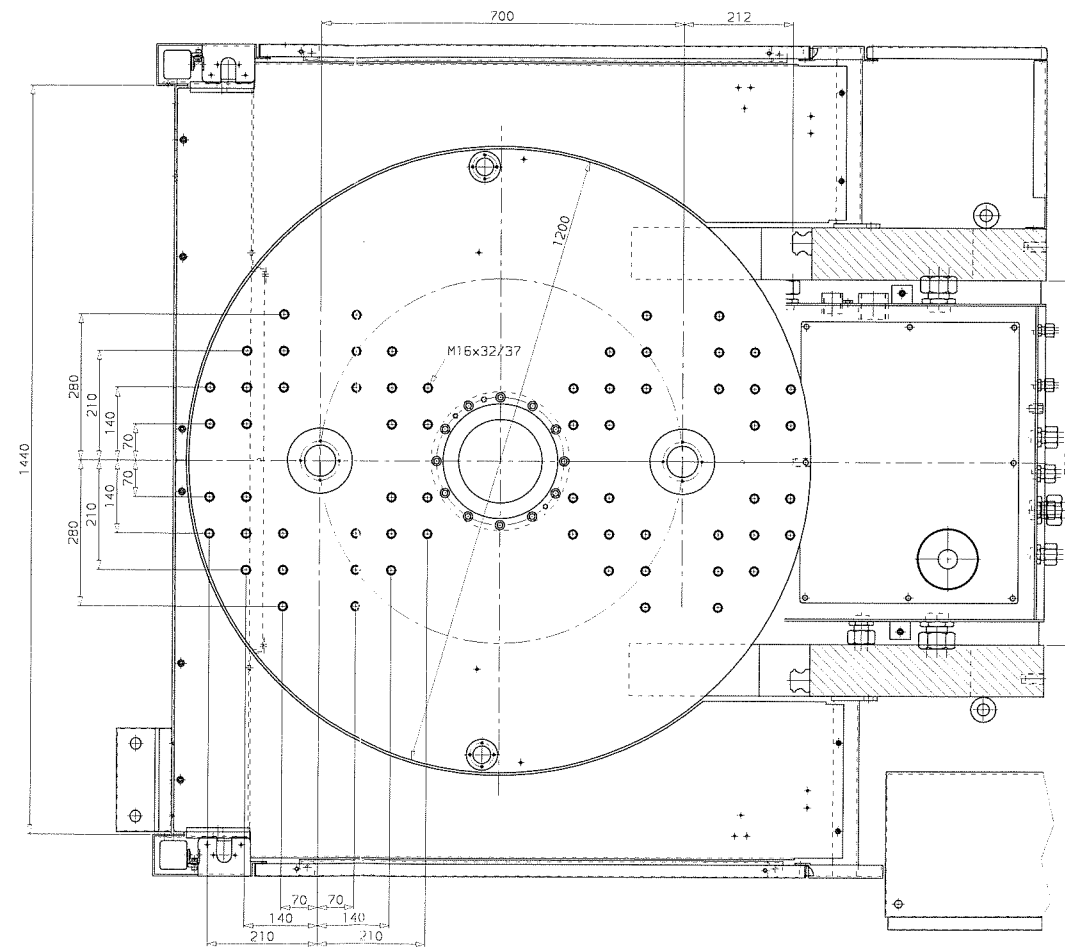
Schnitt A-A
