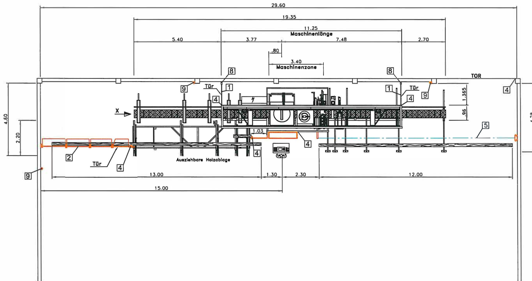
Ansicht X
