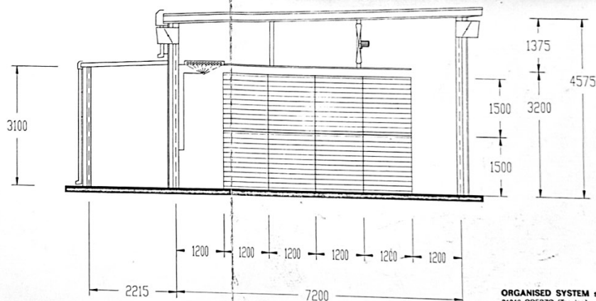
SEZIONE TRASVERSALE ESSICCATOIO
