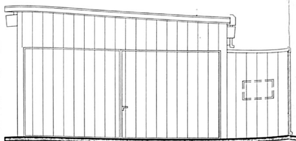
PROSPETTO FRONTALE
