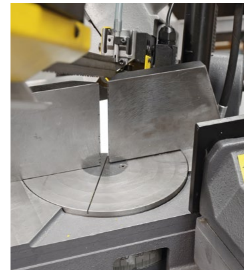
Die Maschine verfügt über einen runden Auflagetisch, der bei Gehrungsschnitten mit dreht. Dadurch gibt es keine Einschnitte in die Auflagefläche
