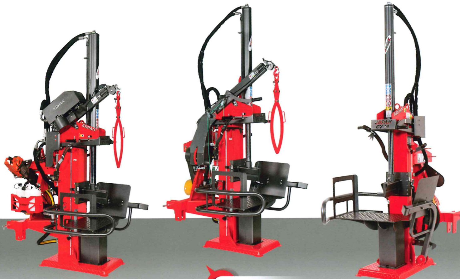
Holzspalter CV mit mechanischer Winde
