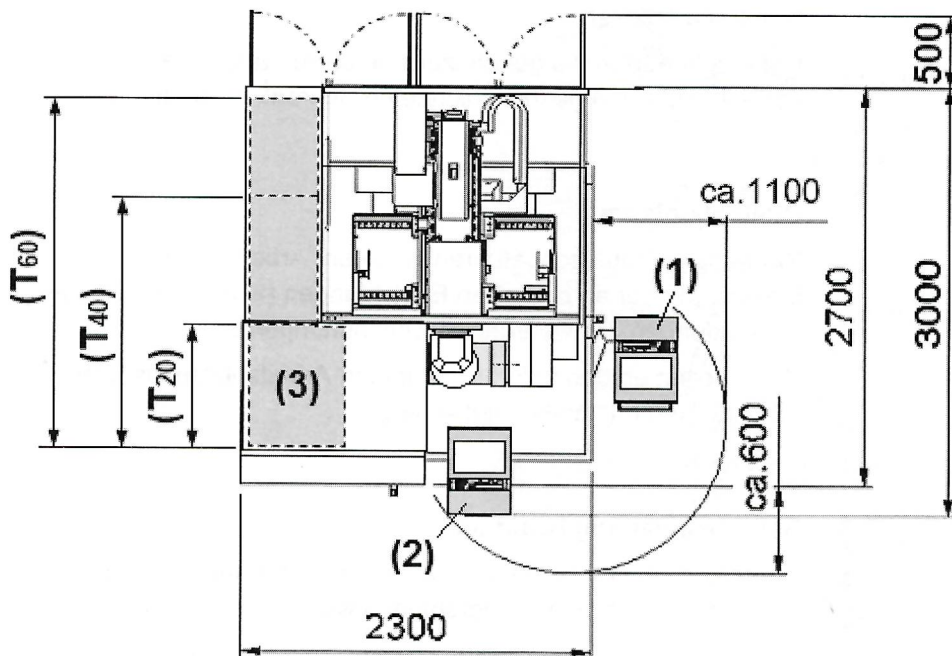
Abb. 6 Maßblatt WF 650 - SEITE
