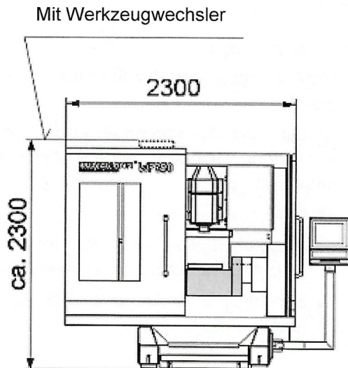
Abb. 5 Maßblatt WF 650 - FRONT
