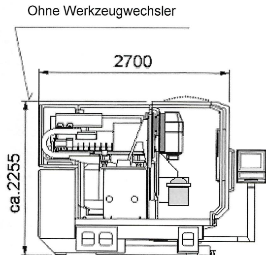
Abb. 6 Maßblatt WF 650 - SEITE
