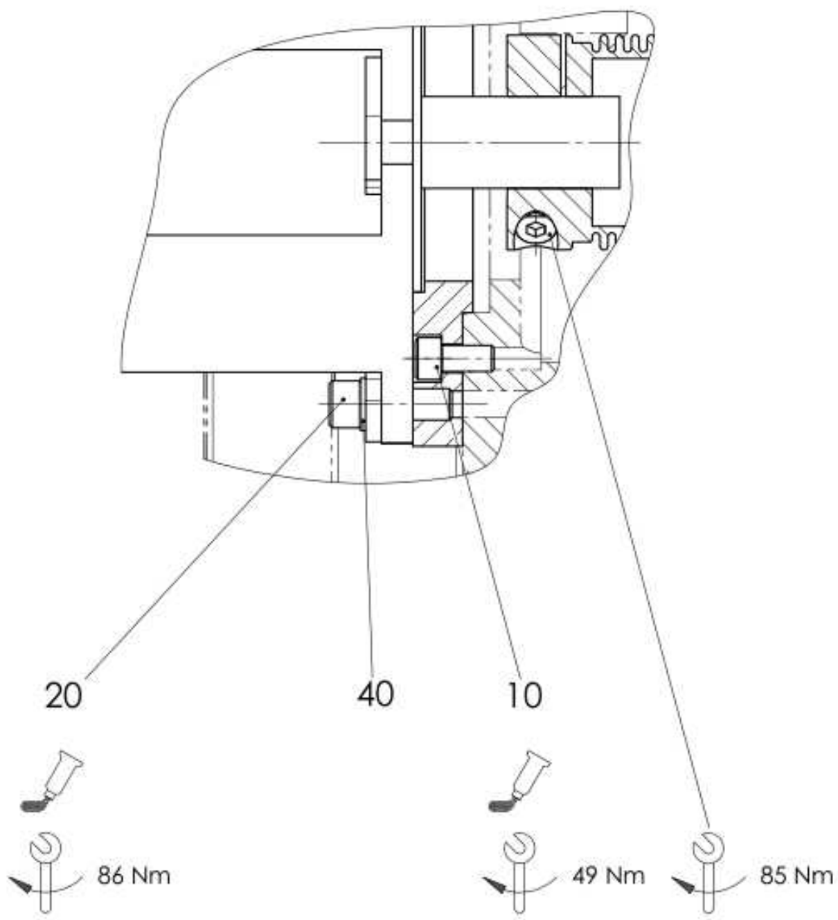
B-B 1:2
